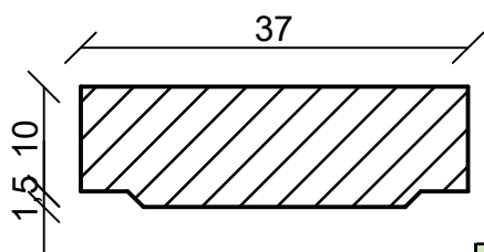
Keresztmetszet
