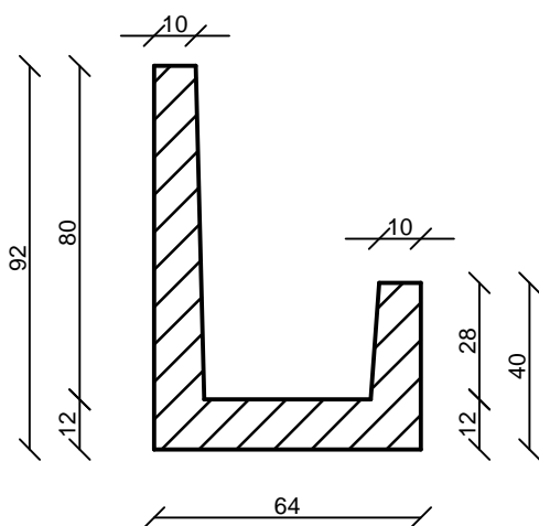
Keresztmetszet
