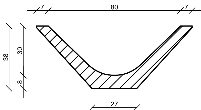
Keresztmetszet
