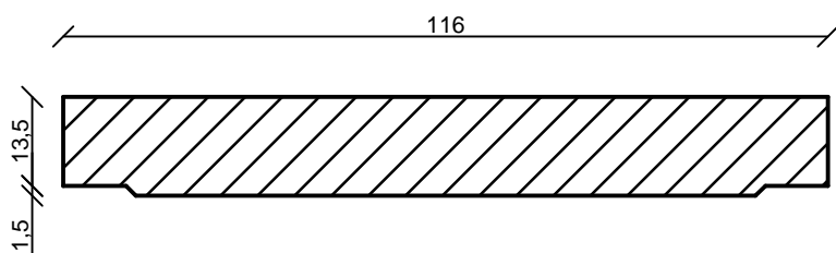
Keresztmetszet
