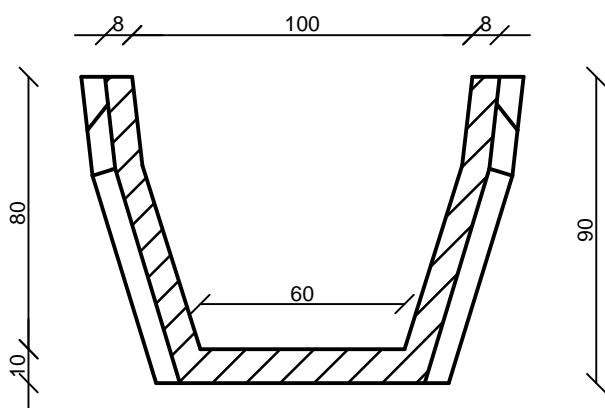
Keresztmetszet
