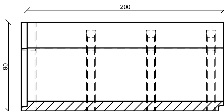
Hosszmetszet
