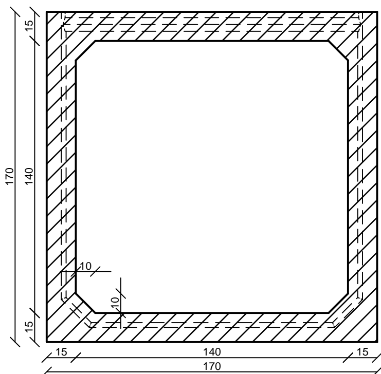
Keresztmetszet
