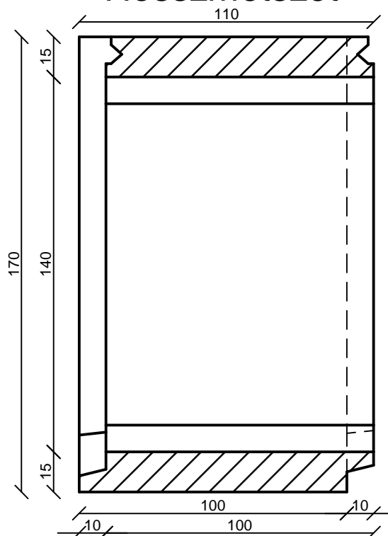
Hosszmetszet
