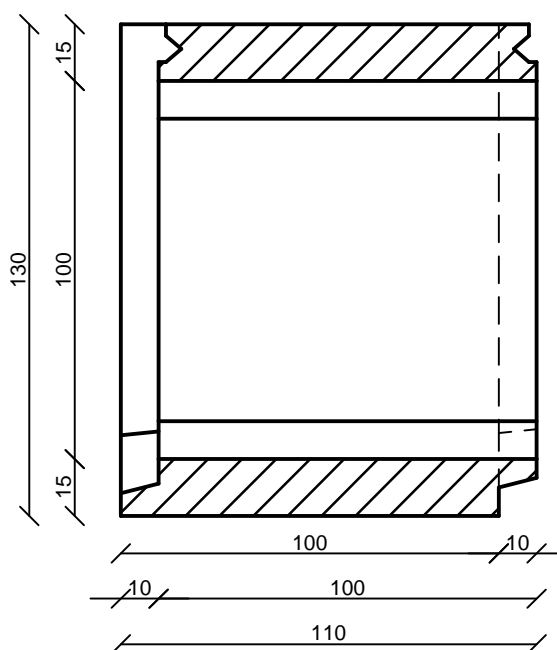
Hosszmetszet
