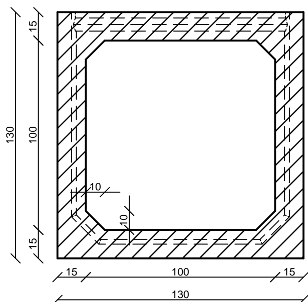
Keresztmetszet
