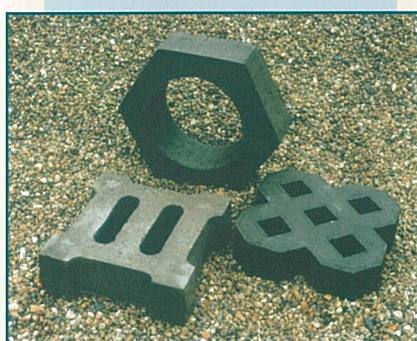
Gyephézagos burkolók és rézsüburkoló elem
