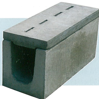
Folyóka elem felül beömlő fedlappal
